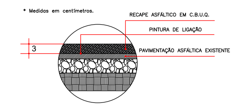
Detalhamento da Pavimentação
